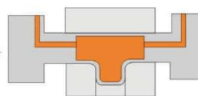
Bulge-Forming液压成型
