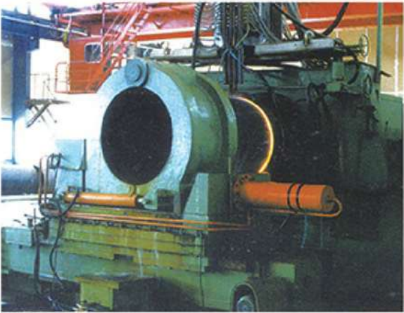
弯管机 Bend machine
