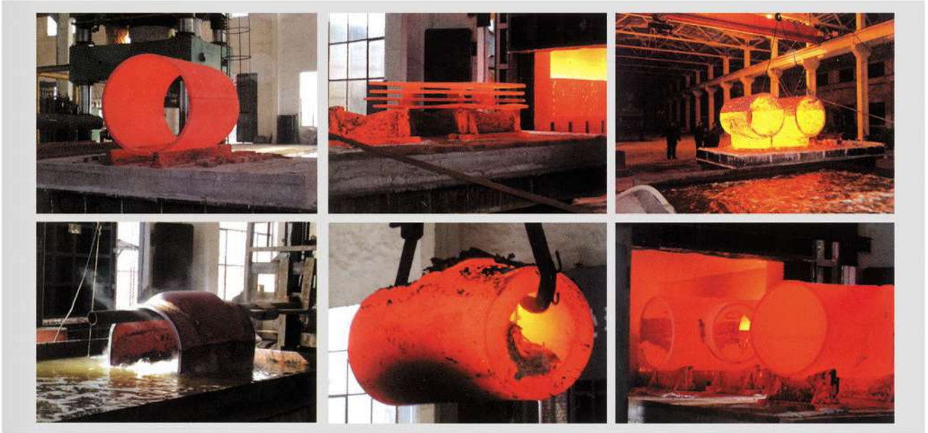
管件热处理 Pipe heat treating
